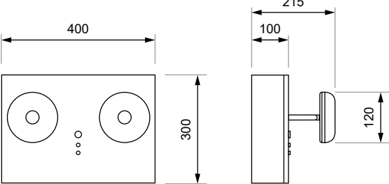
Proyector de dos focos al frente
