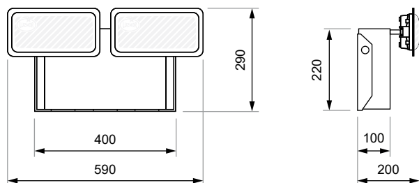
Proyector de dos focos IP42
