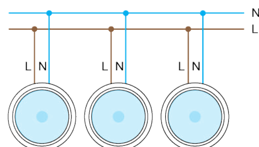
Piloto de balizamiento Élite con difusor opal o transparente.
