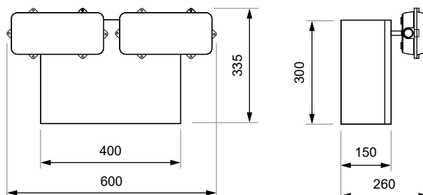
Proyector de dos focos IP66
