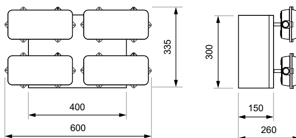
Proyector de cuatro focos IP66
