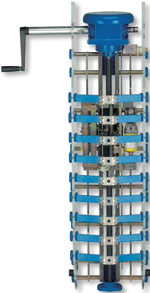
Conmutador en Carga
